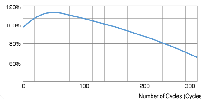
Количество циклов/Емкость
