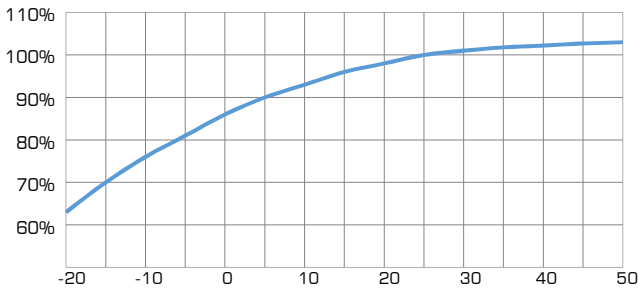
Влияние температуры на емкость
